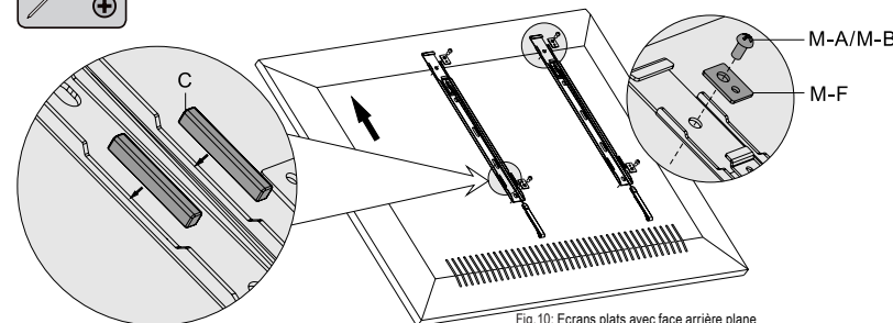
Fig.10: Ecrans plats avec face arrière plane
