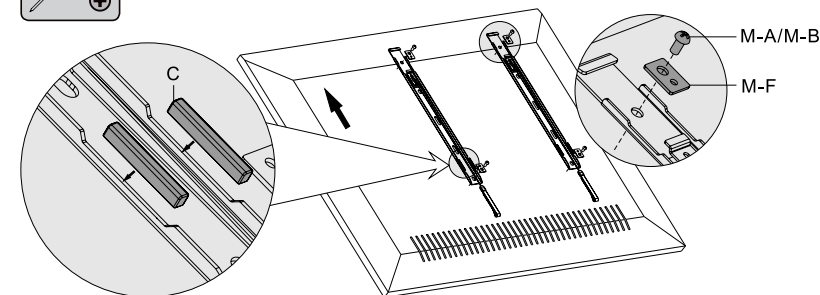
Fig. 2: Flachbildschirme mit flacher Rückseite
