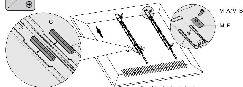
Fig. 14: Schermi piatti con fondo piatto
