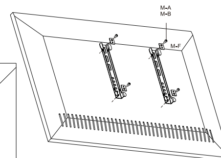
Fig. 2: Flachbildschirme mit flacher Rückseite
