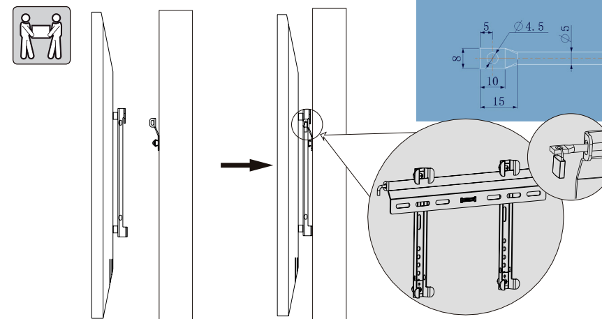
Fig. 13: Assembler et fixer l'écran plat
